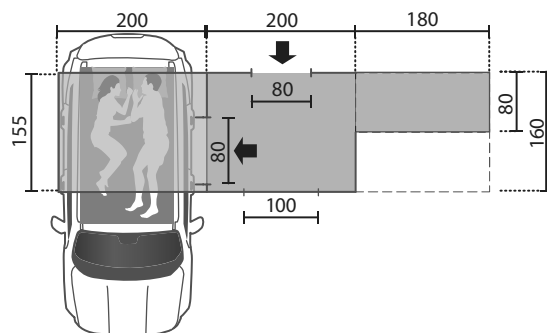
VERANDA INDIPENDENTE 4x4 Art. M/06A
