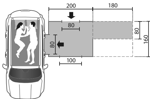
VERANDA INDIPENDENTE Art. M/05A
